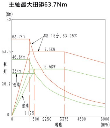
5.5Kw主轴功率扭矩曲线图
